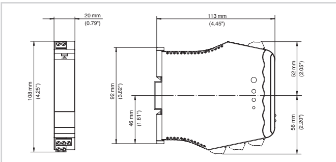
VEGATOR 141 的尺寸
