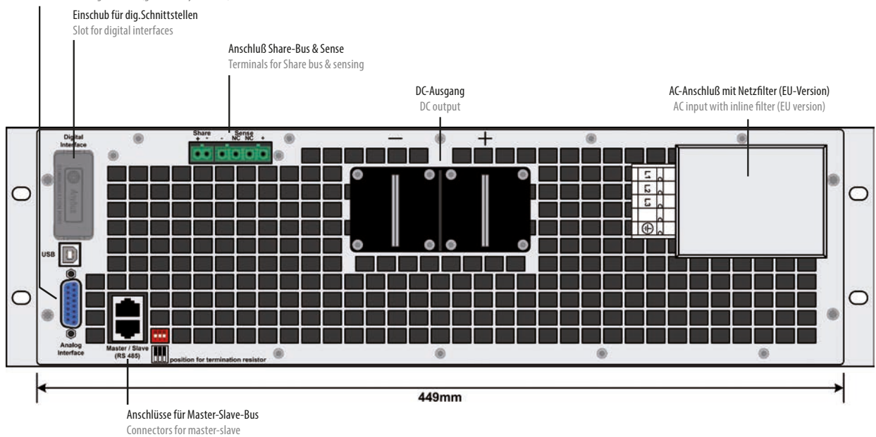
Rückansicht Standardmodell
