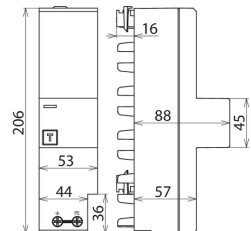
Dimensions DSH ZP B TT 255
