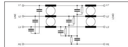
Prinzipschaltbild / Schematic circuit
