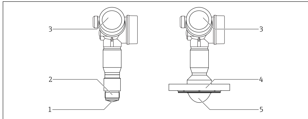
1 Aufbau des Micropilot FMR62
