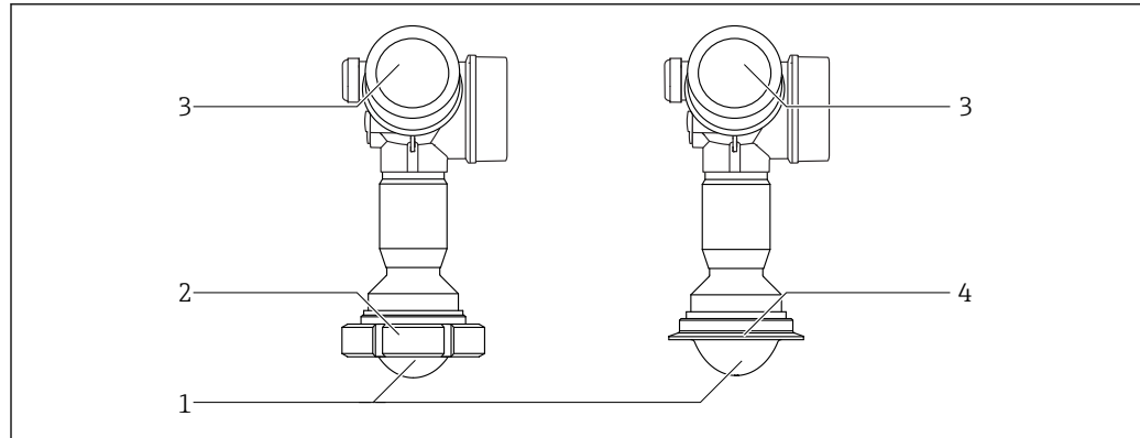
2 Aufbau des Micropilot FMR62
