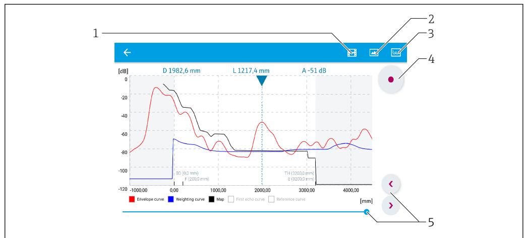
28 Hüllkurvendarstellung (Beispiel) in SmartBlue bei Android
