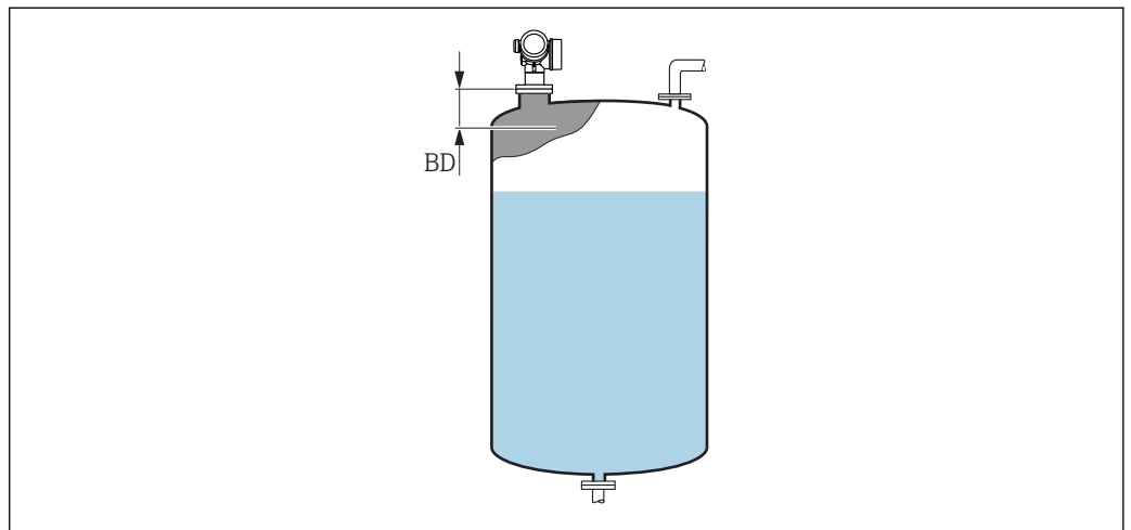
39 Blockdistanz (BD) bei Messung in Flüssigkeiten
