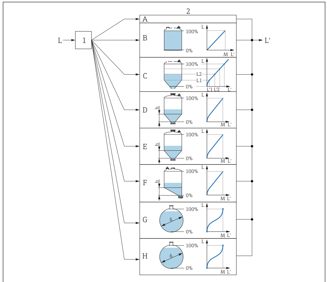
41 Linearisierung: Umrechnung des Füllstands in ein Volumen oder ein Gewicht; die Umrechnung ist von der Behälterform abhängig
