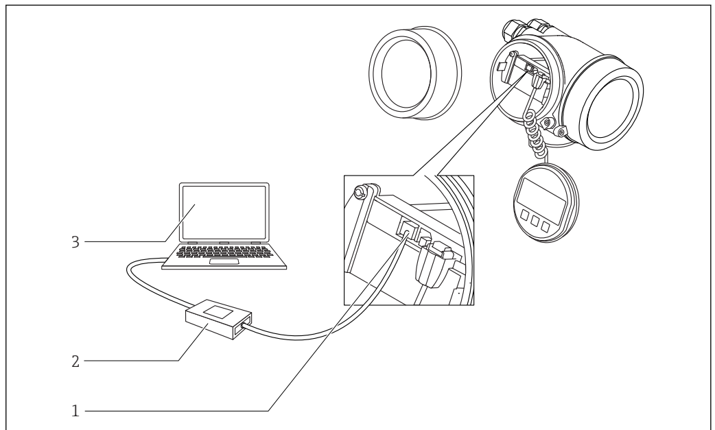
20 DeviceCare/FieldCare über Service-Schnittstelle (CDI)
