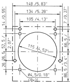
Lochbild Eintrittsfilter Cut-out inlet filter Découpe pour filtre d'entrée
