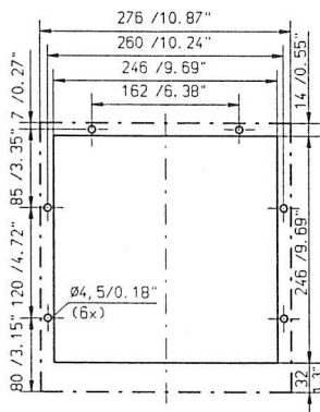
Lochbild Eintrittsfilter/Cut-out inlet filter Découpe filtre d'entrée
