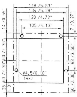
Lochbild Eintrittsfilter Cut-out inlet filter Découpe pour filtre d'entrée
