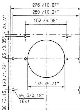
Lochbild Eintrittsfilter/Cut-out inlet filter Découpe filtre d'entrée
