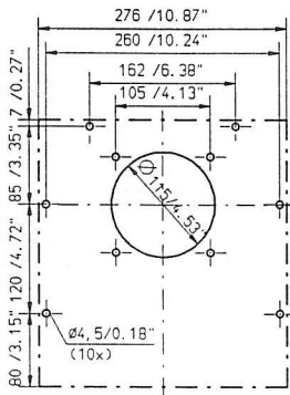
Lochbild Filterlüfter/Cut-out filter fan Découpe ventilateur à filtre 330 m³/h
