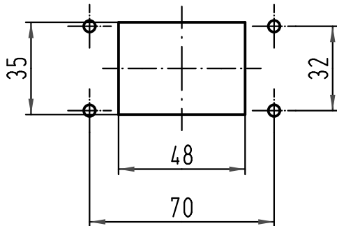
Montageausschnitt 1:2 panel cut out 1:2
