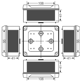
Gehäusewände
