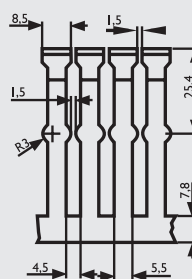
Bauhöhe 60
