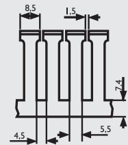
Bauhöhe 40
