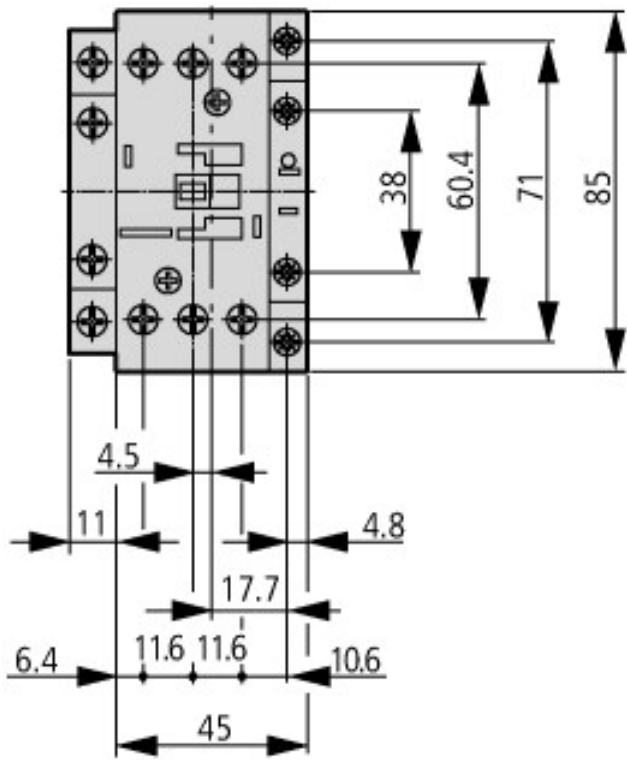
Contacteur avec module de contact auxiliaire
