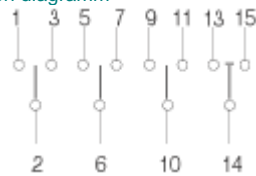
Schaltbild Connection diagram
