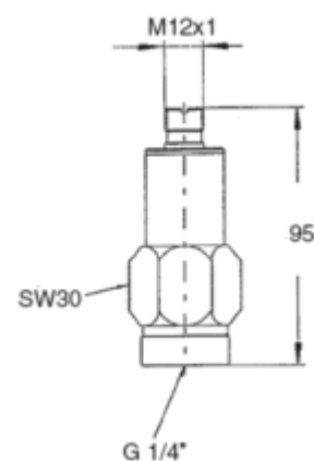
Drucksensor ZDS
