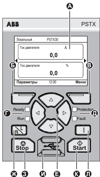
Рис. 3. Панель управления
