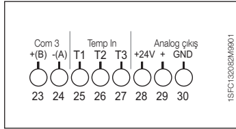
Şekil 2: Terminal bağlantısı
