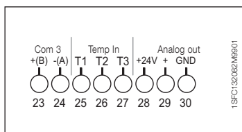
Obrázek 2: Připojení svorek
