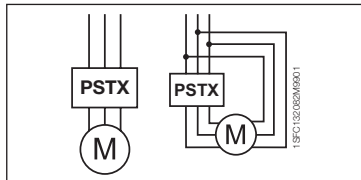
Şekil 1: Direkt, Üçgen
