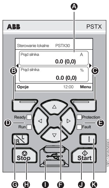
Rysunek 3. Interfejs HMI
