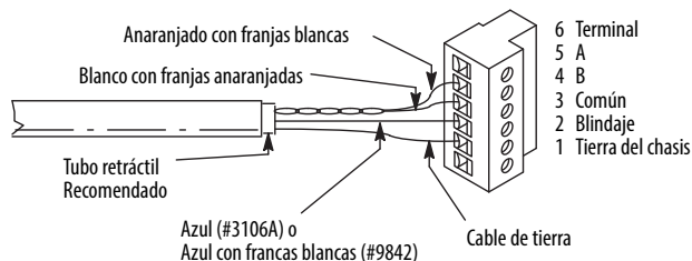
Figura 22 – Conexión de múltiples cables
