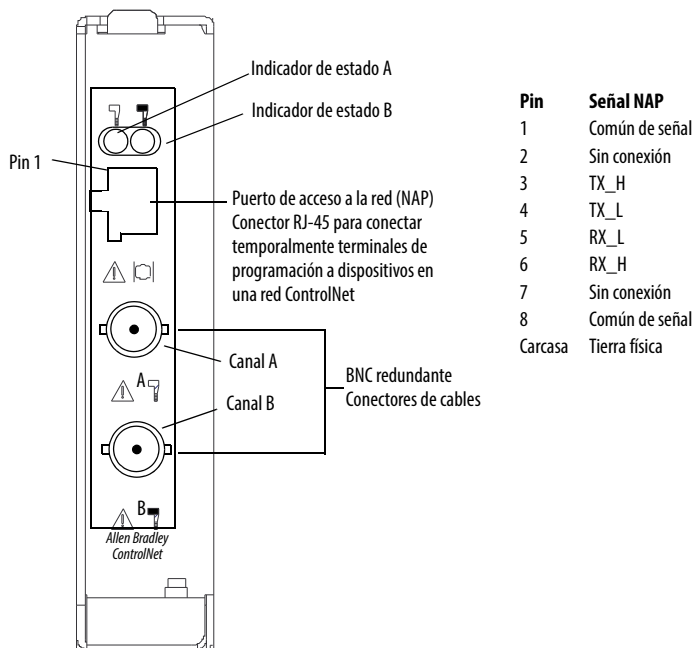
Figura 24 – N.º Módulo de comunicación 2711P-RN155 o 2711P-RN155K
