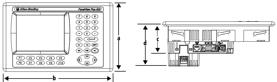
Figura 7 – PanelView Plus 6 – Teclado o teclado/pantalla táctil 600
