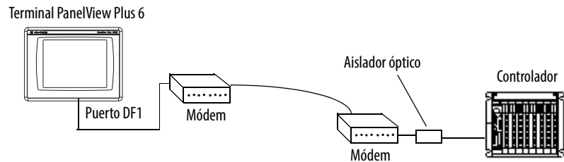
Figura 17 – Conexión de módem
