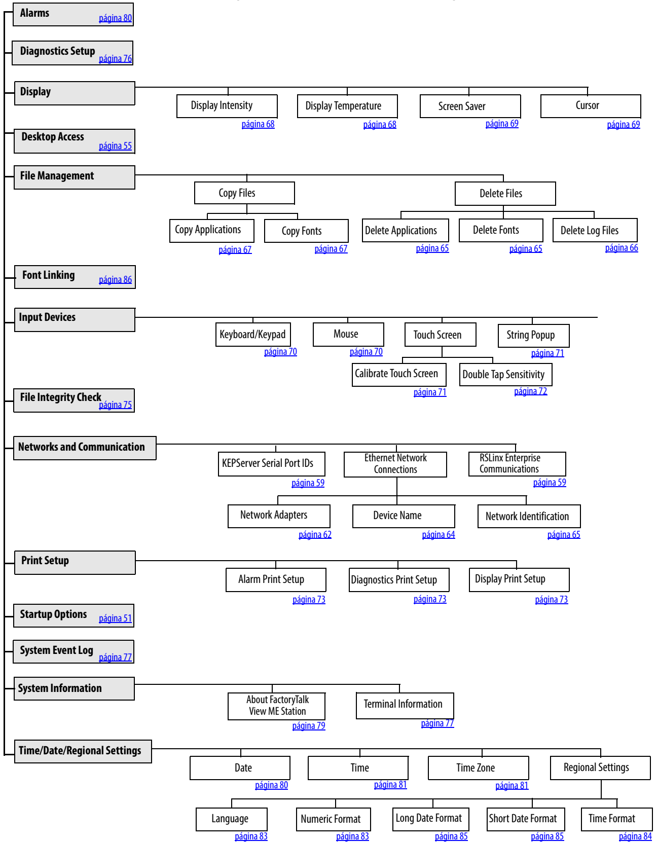
Figura 12 – Estructura del menú Terminal Settings
