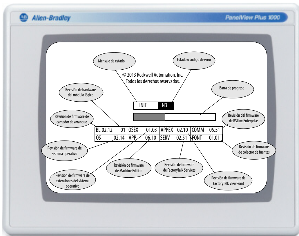
Figura 26 – Pantalla de presentación de puesta en marcha
