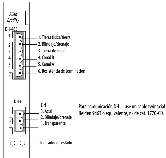
Figura 19 – Conectores del módulo de comunicación DH-485/DH+
