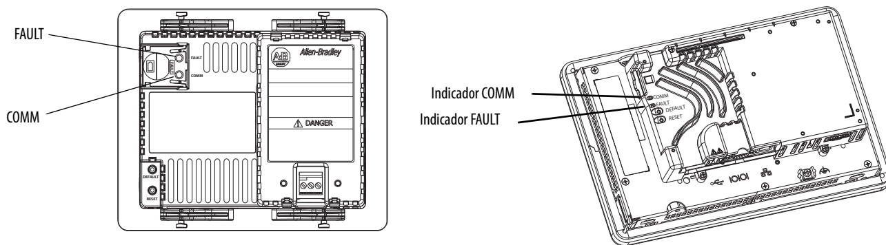
Figura 25 – Indicadores de estado
