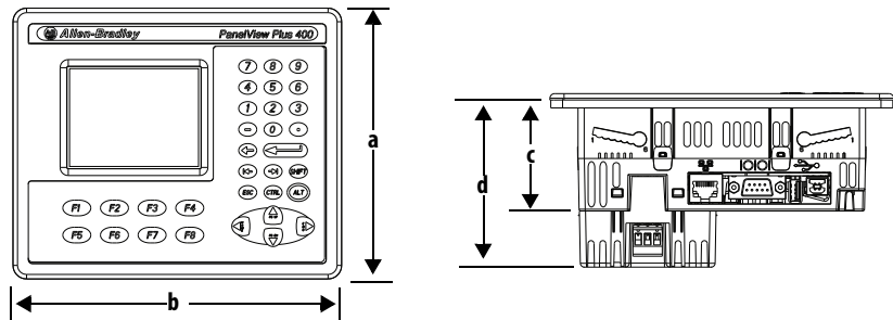
Figura 6 – PanelView Plus 6 – Pantalla táctil 600
