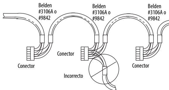
Figura 20 – Conexión en cadena
