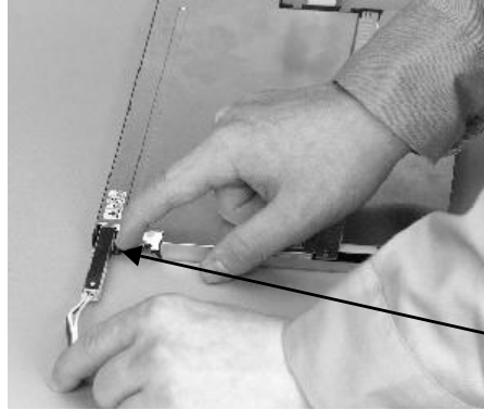
Lengüeta de retención de la luz de retroiluminación
