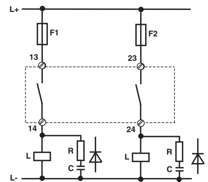
Fig. 5: Extinción de chispas / Spegnimento dell'arco / Vonkdooving
