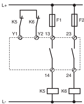
Fig. 3: Excitación bicanal; 2 S / Comando a due canali; 2 S / Tweekanalige aansturing; 2 S
