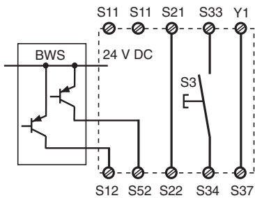
Fig. 8: Control de barrera fotoeléctrica, bicanal, detección de corto circuito transversal mediante BWS, rearme supervisado/Controllo barriera fotoelettrica, bicanale, rilevamento del cortocircuito trasversale mediante fotocellula, start controllato/Tweekanalige lichtscherm-bewaking, detectie van onderlinge sluiting door lichtscherm, bewaakte start
