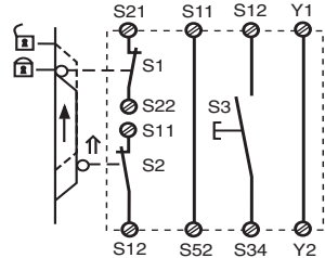
Fig. 6: Schutztürsteuerung zweikanalig, Querschlusserkennung/Two-channel safety gate control, short-circuit recognition/Surveillance de protecteur, commande par 2 canaux, détection des c.c.
