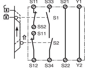
Fig. 7: Schutztürsteuerung zweikanalig, automatischer Start/Two channel safety gate control, automatic reset/Surveillance de protecteur, commande par 2 canaux, validation automatique
