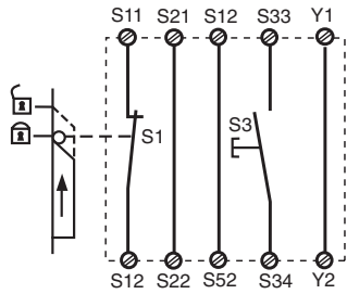
Fig. 5: Control de puerta protectora monocanal/Controllo monocanale riparo mobile/Schermeurbediening éénkanalig
