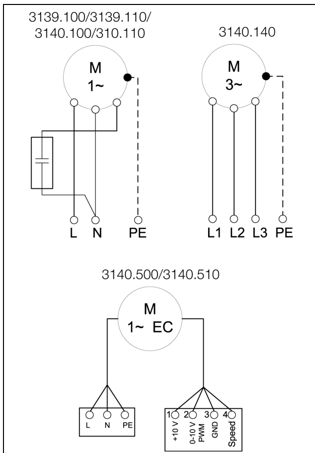
Imagen 2: Esquemas de conexión
