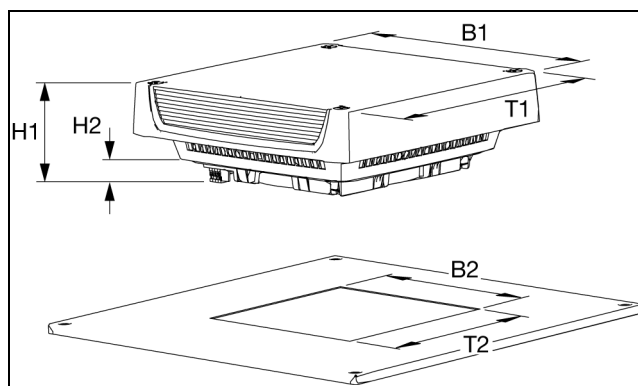
Imagen 5: Dimensiones
