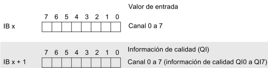
Figura 4-1 Espacio de direcciones del DI 8x24VDC ST con información de calidad
