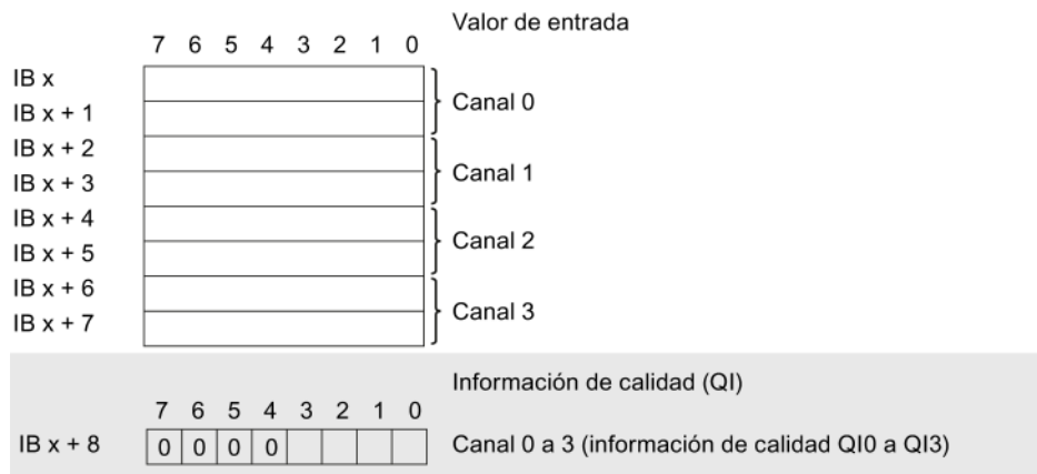
Figura 4-2 Espacio de direcciones del AI 4xI 2-/4-wire ST con información de calidad
