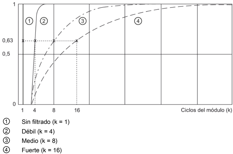
Figura 4-1 Filtrado para AI 4xI 2-/4-wire ST
