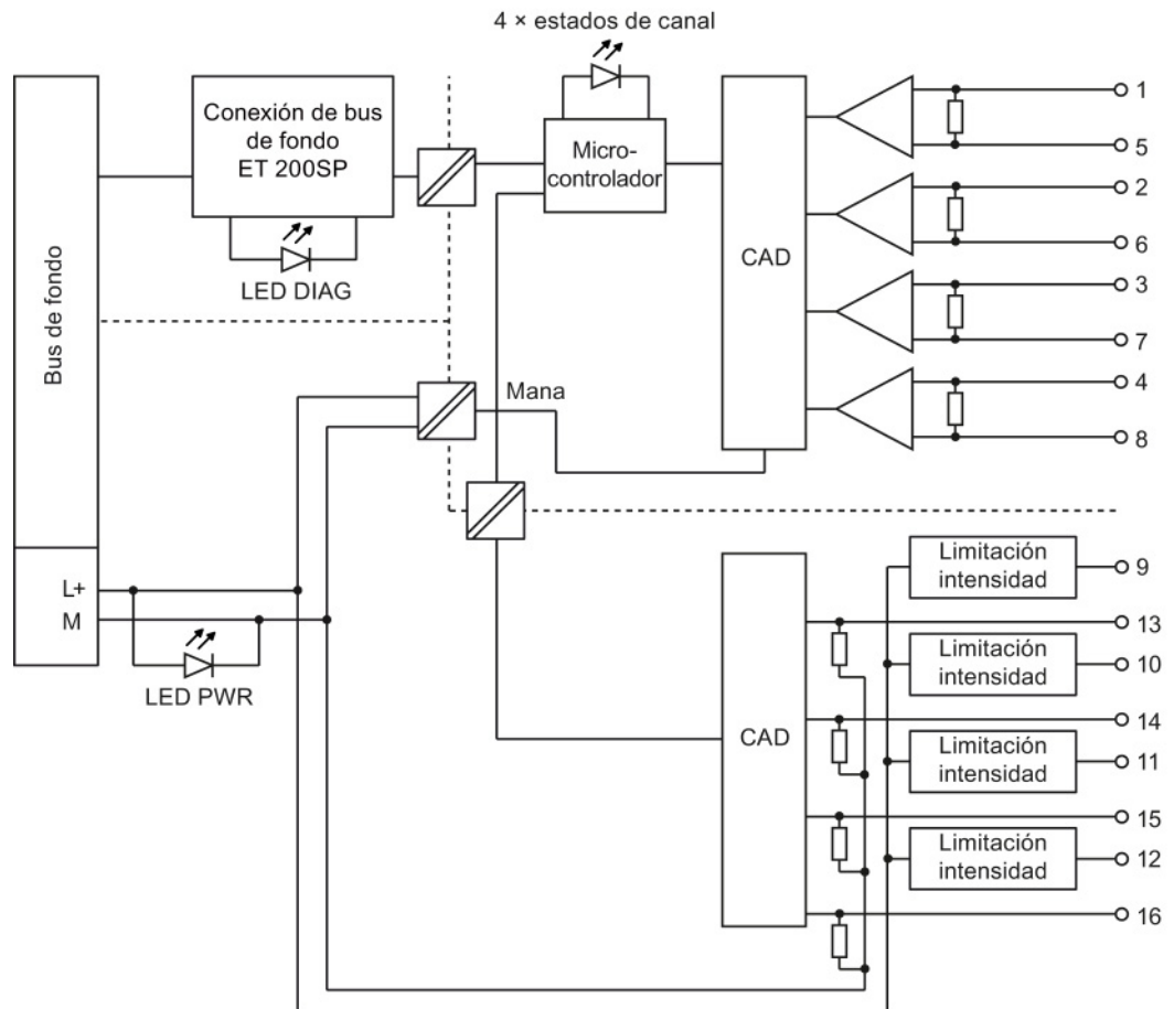
Figura 3-1 Esquema de principio AI 4x1 2-/4-wire ST
