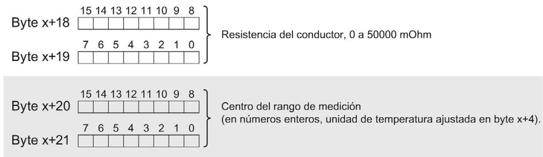
Figura A-3 Estructura de los bytes x a x+21 para los canales 0 a 7
