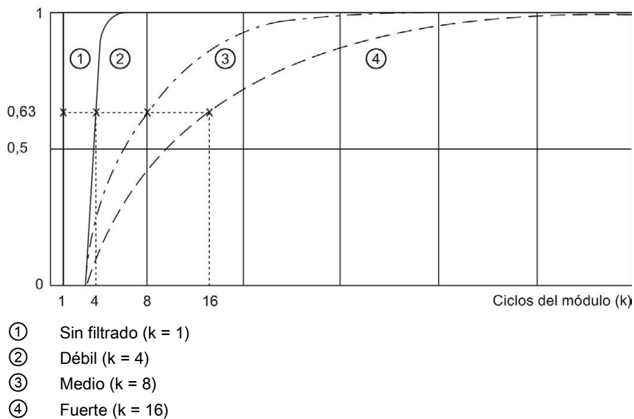
Figura 4-3 Filtrado para AI 8xRTD/TC 2-wire HF
