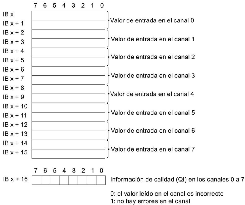
Figura 4-9 Área de direcciones del AI 8×RTD/TC 2-wire HF con información de calidad
