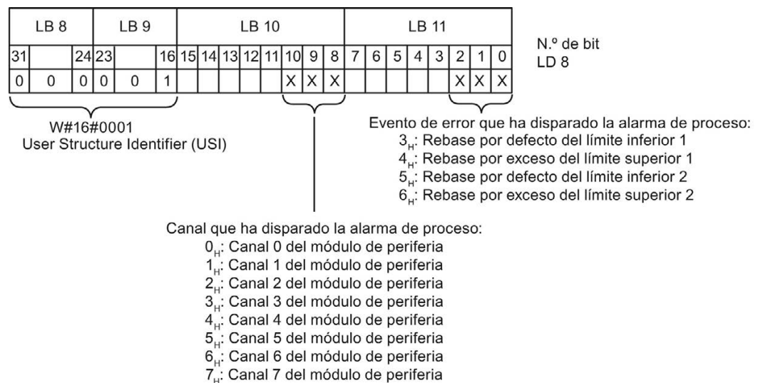
Figura 5-2 Información de arranque del bloque de organización
