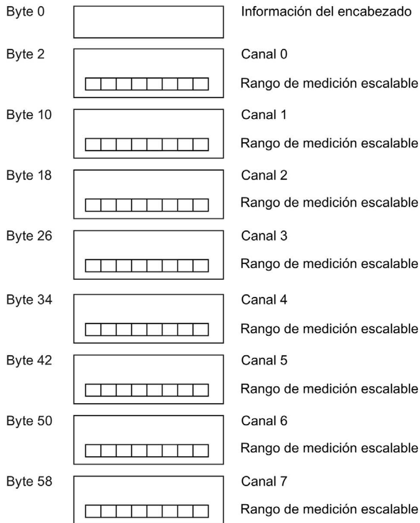
Figura 4-6 Estructura del registro 235
