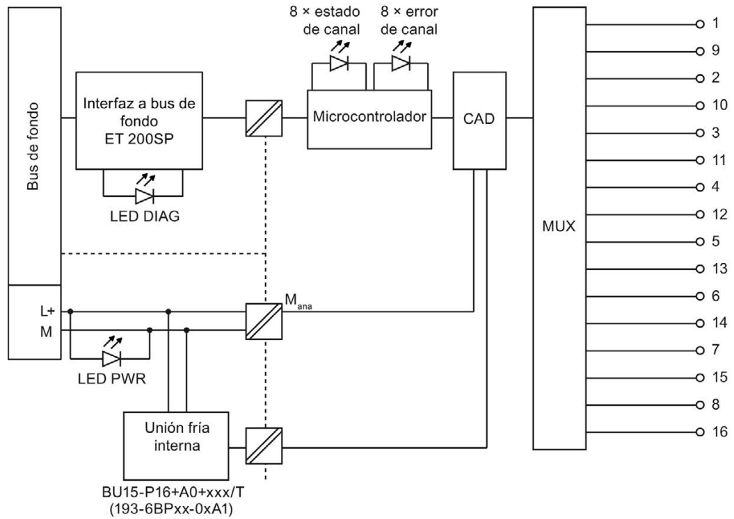
Figura 3-1 Esquema de principio del AI 8xRTD/TC 2-wire HF
