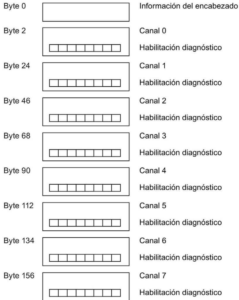
Figura A-1 Estructura del registro 128
