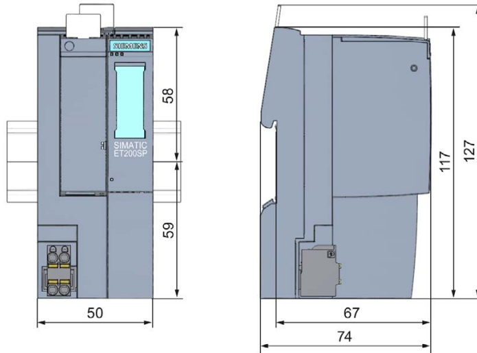
Figura A-1 Croquis acotado del módulo de interfaz IM 155-6 PN ST (vista frontal y lateral)
