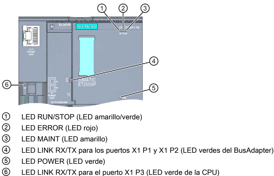
Figura 4-1 Indicadores LED de CPU y BusAdapter
