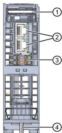
Figura 2-4 Vista de la CPU 1511-1 PN (sin tapa frontal), lado anterior
