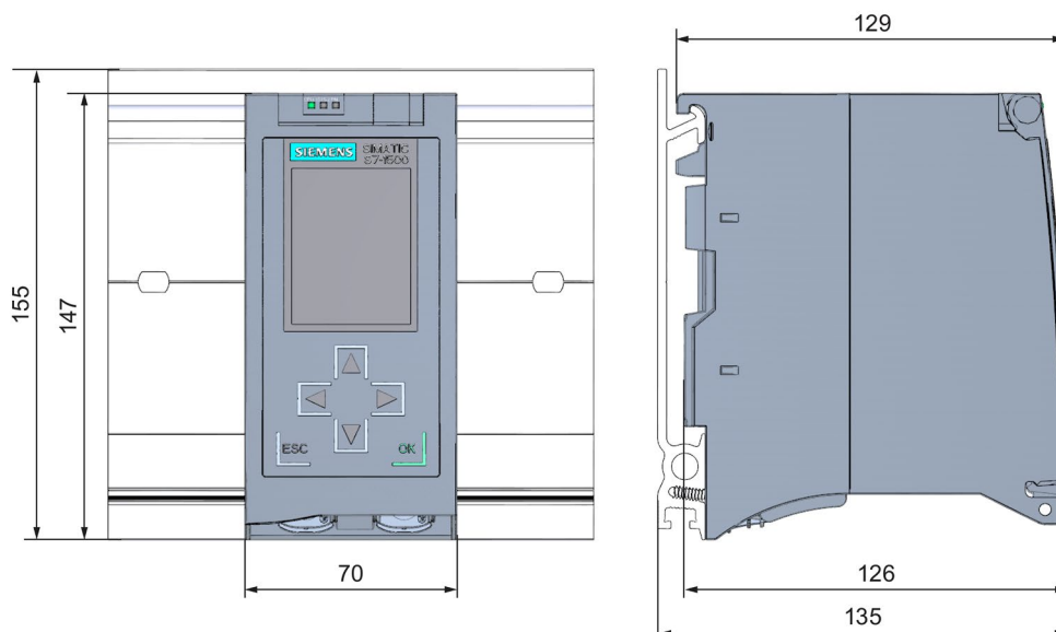
Figura A-1 Croquis acotado de la CPU 1515-2 PN, vista frontal y lateral
