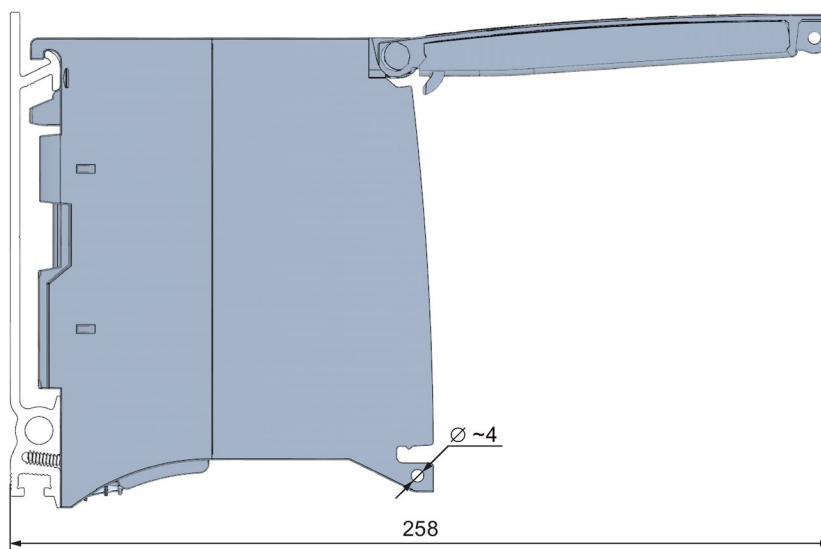
Figura A-2 Croquis acotado de la CPU 1515-2 PN, vista lateral con tapa frontal abierta
