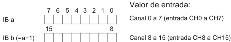
Figura 4-1 Espacio de direcciones en la configuración como DI 16x24VDC BA de 1 x 16 canales
