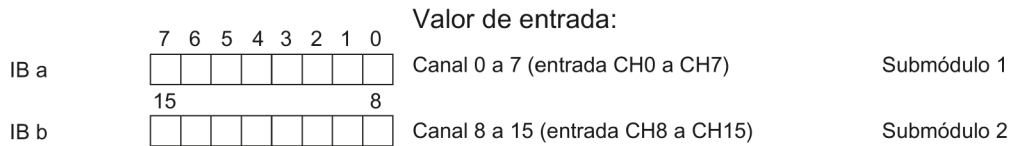
Figura 4-2 Espacio de direcciones en la configuración como DI 16x24VDC BA S de 2 x 8 canales
