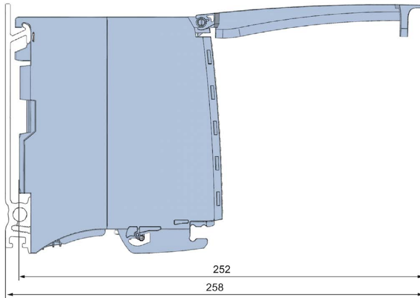
Figura A-2 Croquis acotado del módulo DI 16x24VDC BA, vista lateral con tapa frontal abierta
