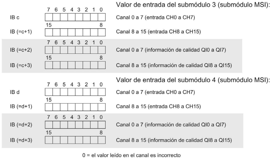
Figura 4-4 Espacio de direcciones en la configuración como DI 16x24VDC BA MSI de 1 x 16 canales con información de calidad
