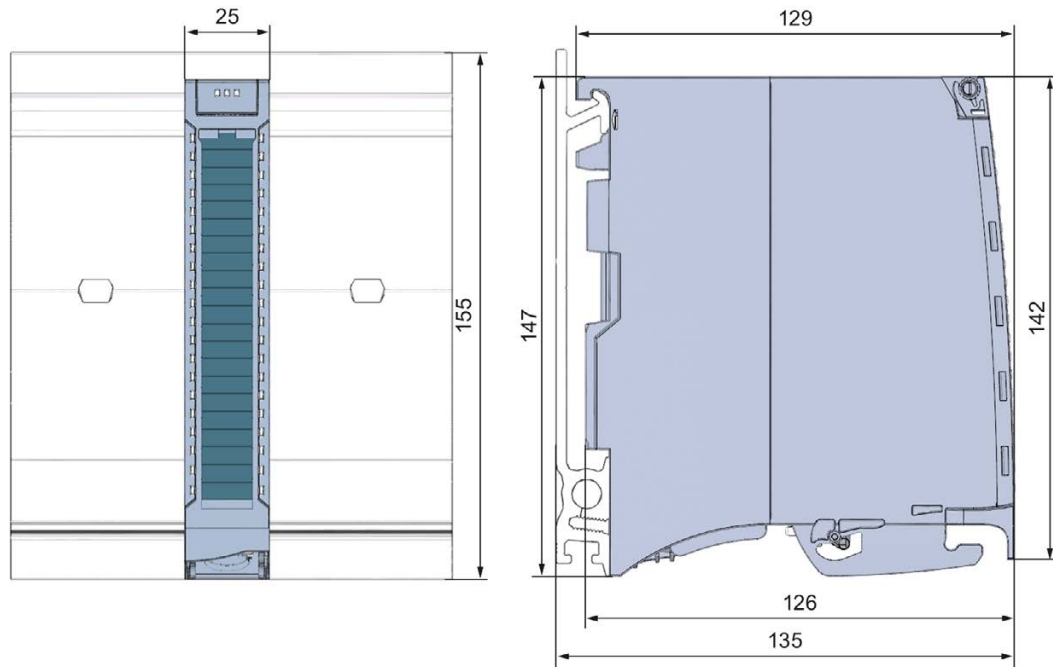
Figura A-1 Croquis acotado del módulo DI 16x24VDC BA
