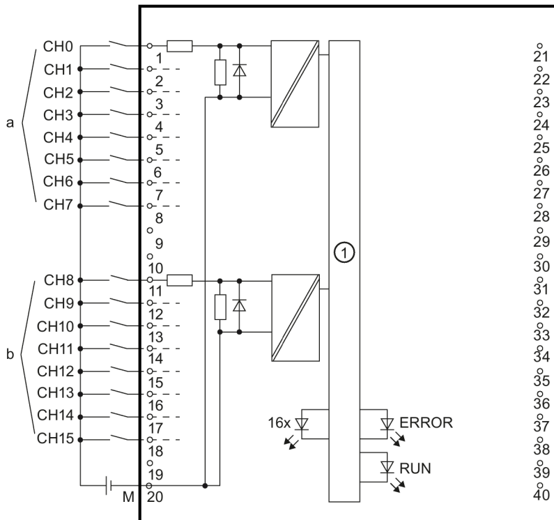
Figura 3-1 Esquema de principio y asignación de conexiones
