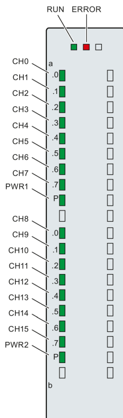
Figura 5-1 LED del módulo DQ 16x24VDC/0.5A BA
