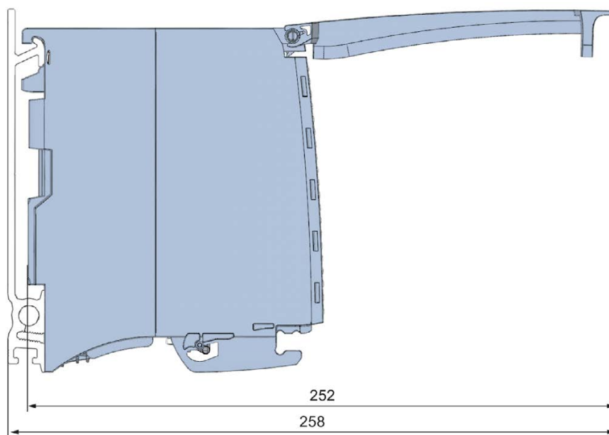
Figura A-2 Croquis acotado del módulo DQ 16x24VDC/0.5A BA, vista lateral con tapa frontal abierta
