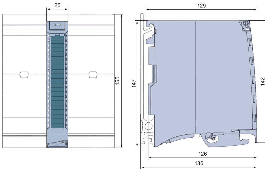
Figura A-1 Croquis acotado del módulo DQ 16x24VDC/0.5A BA
