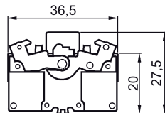
Imagen 5-60 3SB3400-1A, 3SB3400-1D, 3SB3400-1C, 3SB3400-1B
