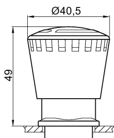
Imagen 5-32 3SB3110-1HA20
