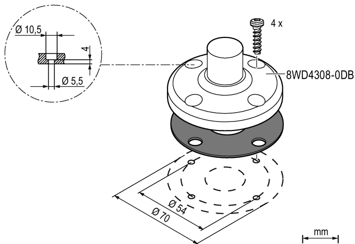
8WD4308-0DB = pata suelta, plástico, para montaje en tubo
