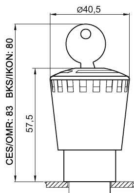
Imagen 5-34 3SB3110-1KA20 (CES), 3SB3110-1LA20 (BKS), 3SB3110-1MA20 (OMR)
