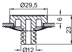
Imagen 5-55 3SB1902-0AQ
