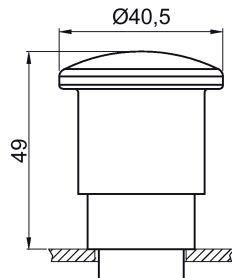
Imagen 5-48 3SB3500-1TA20
