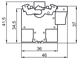
Imagen 5-61 3SB3400-1F, 3SB3400-1G, 3SB3400-1L, 3SB3400-1H
