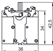
Imagen 5-58 3SB3400-0M
