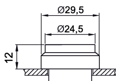
Imagen 5-2 3SB3000-0BA.1
