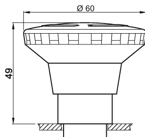
Imagen 5-18 3SB3000-1AA20
