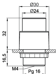
Imagen 5-14 3SB3000-0EA11
