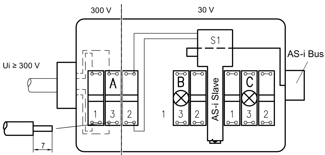
Imagen 6-4 Cableado correcto
