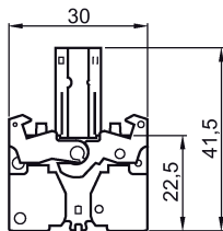
Imagen 5-66 3SB3403-1P., 3SB3403-1Q., 3SB3403-1R.
