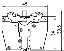
Imagen 5-57 3SB3400-0A
