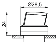
Imagen 5-8 3SB300.-2.A.1
