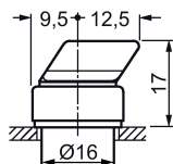
Imagen 4-4 3SB2.0.-2..01
