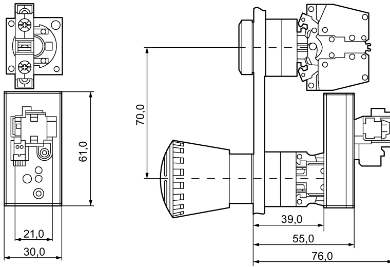
Imagen 6-3 3SF5402-1AA05, 3SF5402-1AB05
