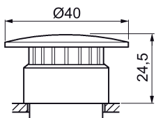
Imagen 5-41 Pulsadores de seta 3SB3500-1GA.1, pulsadores de seta luminosos 3SB3501-1GA.1, interruptores de presión-tracción 3SB3501-1CA.1
