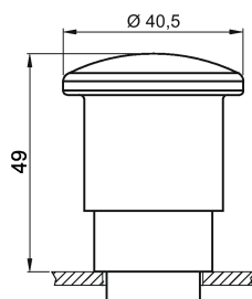
Imagen 5-16 3SB3000-1TA20
