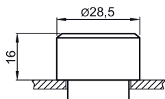
Imagen 5-38 3SB3500-0AA.2
