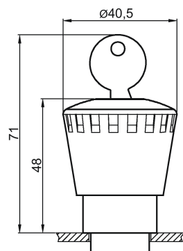
Imagen 5-19 3SB3000-1BA20
