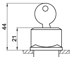
Imagen 5-33 3SB3110-1BA20
