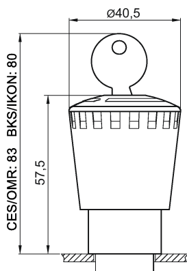
Imagen 5-20 3SB3000-1KA20 (CES), 3SB3000-1LA20 (BKS), 3SB3000-1MA20 (O.M.R.)
