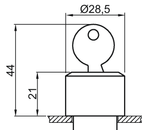
Imagen 5-9 3SB3000-4HD.1
