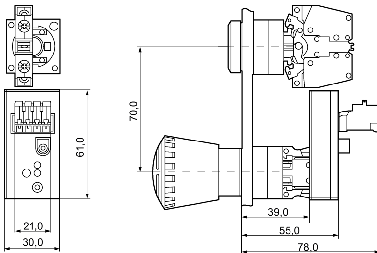
Imagen 6-2 3SF5402-1AA04, 3SF5402-1AB04
