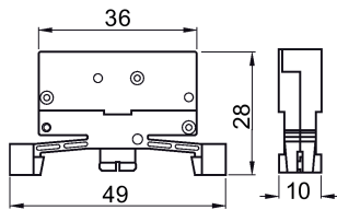
Imagen 5-72 3SB3423-2F, 3SB3423-2G, 3SB3423-2H
