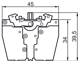
Imagen 5-63 3SB3403-0A, 3SB3403-0H, 3SB3403-0D, 3SB3403-0E
