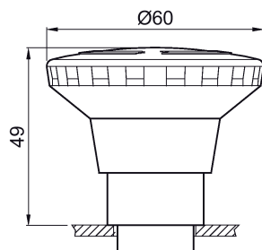
Imagen 5-50 3SB3500-1AA20
