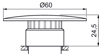
Imagen 5-42 Pulsadores de seta 3SB3500-1QA.1, pulsadores de seta luminosos 3SB3501-1QA.1, interruptores de presión-tracción 3SB3500-1RA.1
