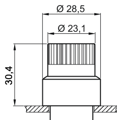
Imagen 5-12 3SB3000-0CA.1
