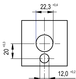
Imagen 5-1 Plantilla de taladros
