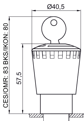
Imagen 5-52 3SB3500-1KA20 (CES), 3SB3500-1LA20 (BKS), 3SB3500-1MA20 (O.M.R.)
