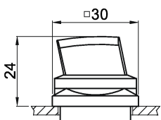
Imagen 5-30 3SB3110-2.A.1
