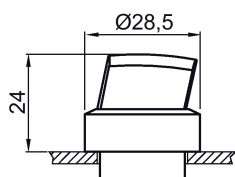
Imagen 5-39 3SB350.-2.A.1
