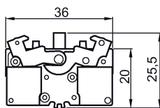
Imagen 5-56 3SB3400-0B, 3SB3400-0C
