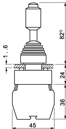
Imagen 5-11 3SB120-7.V01, 3SB1201-7.W20
