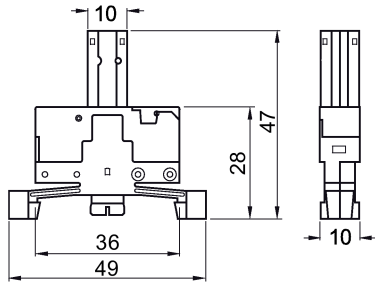
Imagen 5-71 3SB3423-1P, 3SB3423-1Q, 3SB3423-1R
