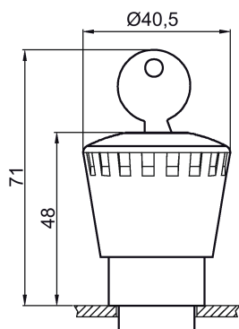
Imagen 5-51 3SB3500-1BA20
