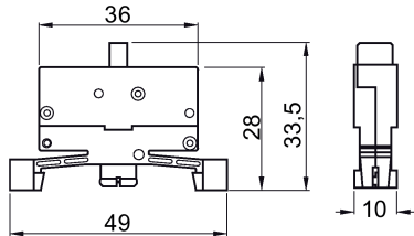
Imagen 5-70 3SB3423-0B, 3SB3423-0C
