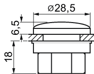
Imagen 5-26 3SB3921-0AA
