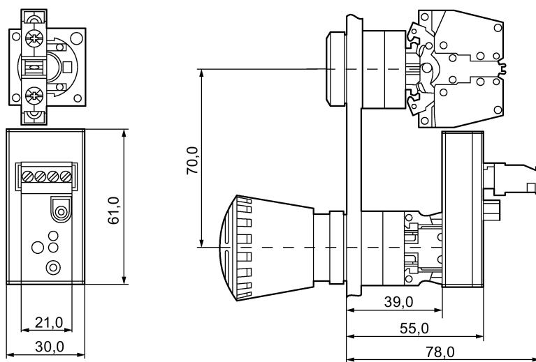
Imagen 6-1 3SF5402-1AA03, 3SF5402-1AB03
