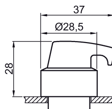
Imagen 5-44 3SB3500-3PA.1
