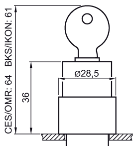
Imagen 5-46 3SB3500-4LD.1 (CES), 3SB3500-5AD.1 (BKS), 3SB3500-3AG.1 (O.M.R)
