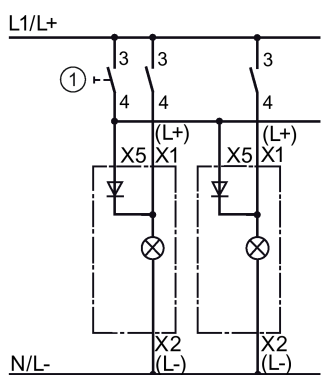
Imagen 5-75 Portalámparas 3SB3400-1L para lámparas incandescentes, máx. 2,6 W, o lámparas LED, AC o DC
