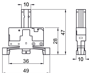
Imagen 5-69 3SB3420-1P., 3SB3420-1Q., 3SB3420-1R.
