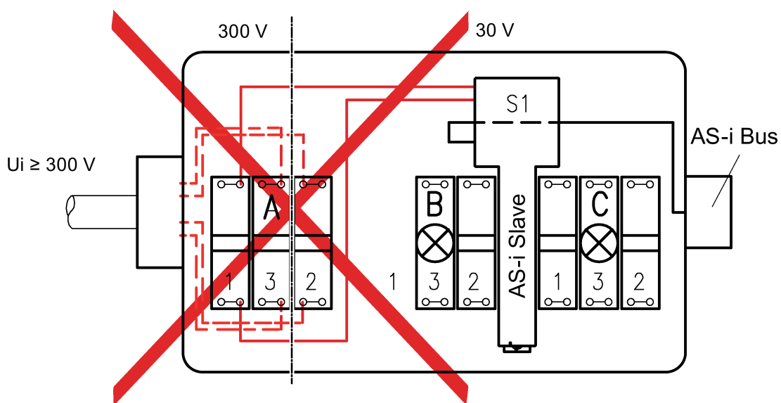
Imagen 6-5 Cableado incorrecto
