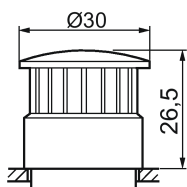
Imagen 5-5 3SB3000-1DA.1
