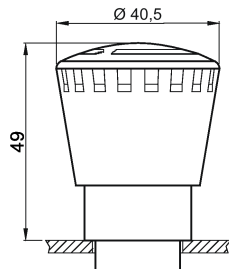
Imagen 5-17 3SB3000-1HA2.
