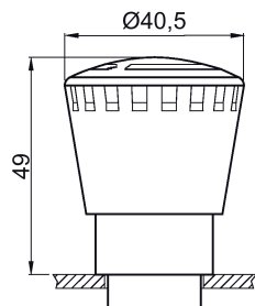
Imagen 5-49 3SB3500-1HA2.
