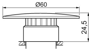
Imagen 5-7 3SB3000-1QA.1
