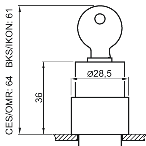
Imagen 5-10 3SB3000-4LD.1 (CES), 3SB3000-4LD05 (CES con vigilancia de llave), 3SB3000-5AD.1 (BKS), 3SB3000-3AG.1 (O.M.R.)
