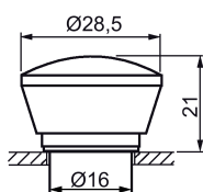
Imagen 4-6 3SB2.0.-1AC01
