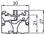
Imagen 5-62 3SB3403-0B, 3SB3403-0C
