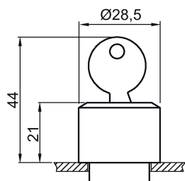
Imagen 5-45 3SB3500-4AD.1
