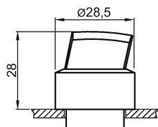
Imagen 5-43 3SB350.-2PA.1
