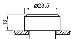
Imagen 5-3 3SB3000-0AA.2
