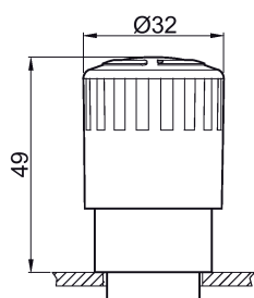
Imagen 5-47 3SB3500-1FA20
