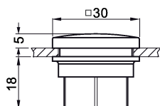
Imagen 5-36 3SB3941-0AA
