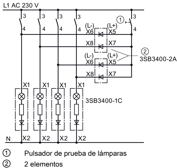
Imagen 5-77 Ejemplo de circuito de prueba de lámparas con elemento 3SB3400-2A
