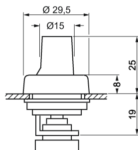
Imagen 5-13 3SB1000-7CH07
