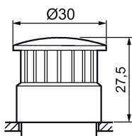
Imagen 5-40 Pulsadores de seta 3SB3500-1DA.1, pulsadores de seta luminosos 3SB3501-1DA.1, interruptores de presión-tracción 3SB3500-1EA.1
