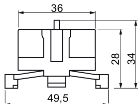
Imagen 5-67 3SB3420-0B, 3SB3420-0C
