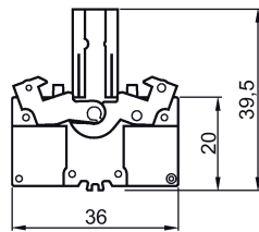
Imagen 5-59 3SB3400-1P., 3SB3400-1Q, 3SB3400-1R
