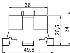
Imagen 5-68 3SB3420-1A, 3SB3420-1C
