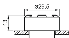
Imagen 5-4 3SB3001-0BA.1
