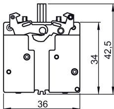
Imagen 5-64 3SB3403-0M
