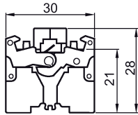
Imagen 5-65 3SB3403-1A, 3SB3403--1C
