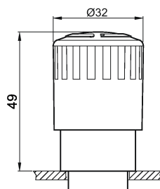
Imagen 5-15 3SB3000-1FA20
