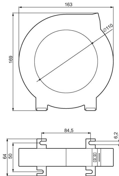
Figura 13-12 3UL2305-1A
