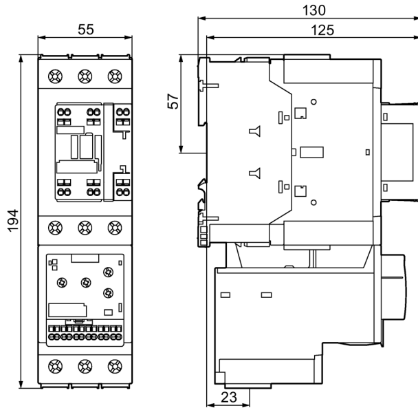
Figura C-11 3RR2143-3A.30 con contactor
