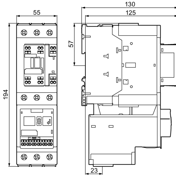
Figura C-15 3RR2243-3F.30 con contactor
