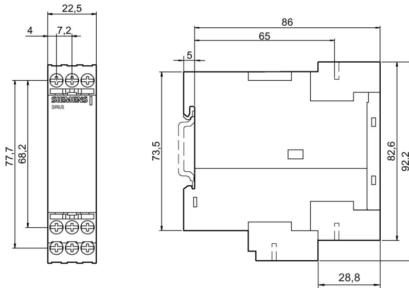
Figura C-19 Relés de monitoreo 3UG4. con 3 bornes de conexión de tornillo
