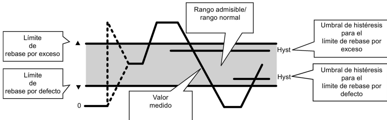
Figura B-1 Explicación de la histéresis
