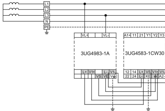
Figura 13-16 Ejemplo de conexión: módulo adaptador - relé de monitoreo de aislamiento
