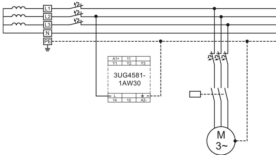
Figura 9-3 Monitoreo de falla a tierra/defectos de aislamiento en una red AC IT de 4 conductores
