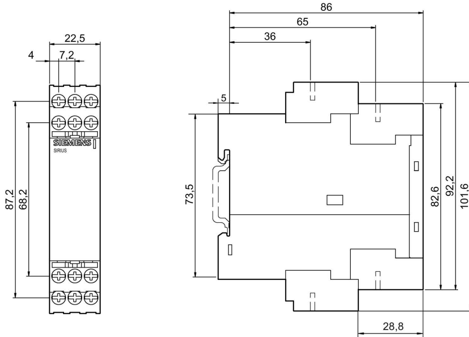
Figura C-21 Relés de monitoreo 3UG4. con 4 bornes de conexión de tornillo
