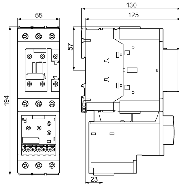
Figura C-9 3RR2143-1A.30 con contactor
