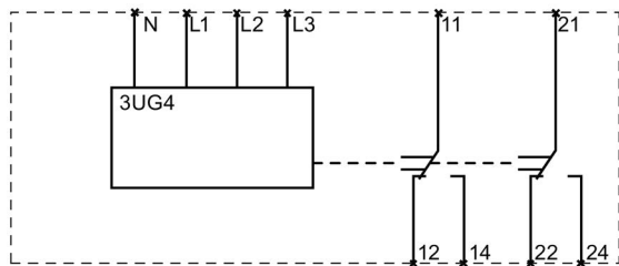
Relé de monitoreo de red 3UG4618
