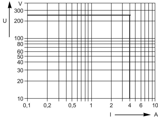
Figura 9-12 Carga AC (ohmica)
