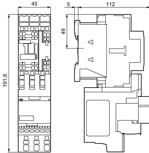
Figura C-7 3RR2.42-2A.30 con contactor
