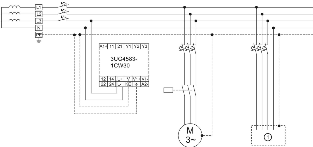
Figura 9-10 Vigilancia de fallas a tierra/defectos de aislamiento en una red AC de 4 conductores
