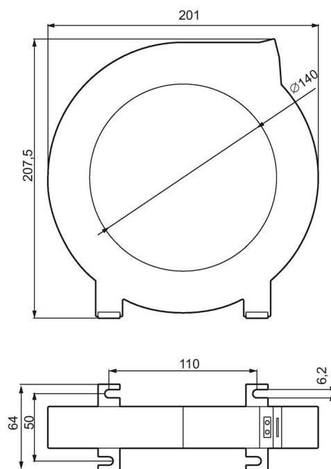
Figura 13-13 3UL2306-1A
