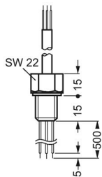
Figura 13-1 Electrodo de alambre tripolar 3UG3207-3A
