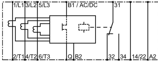
Figura 4-5 1 contacto conmutado, trifásico
