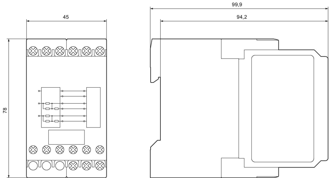
Figura C-25 Módulo adaptador 3UG4983-1A
