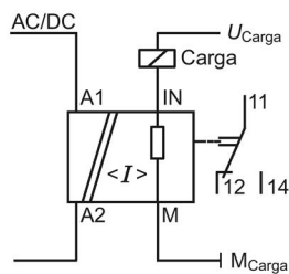
3UG462...-AW30 Modo monofásico
