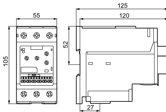
Figura C-12 3RR2143-3A.30 con soporte de conexión para instalación independiente
