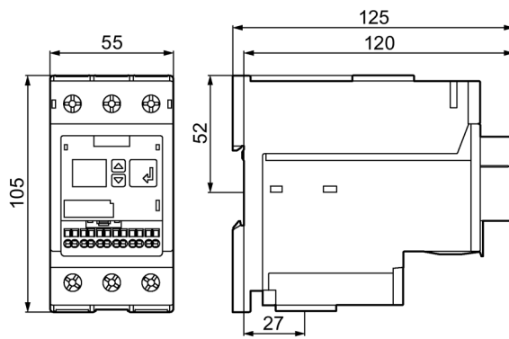
Figura C-16 3RR2243-3F.30 con soporte de conexión para instalación independiente
