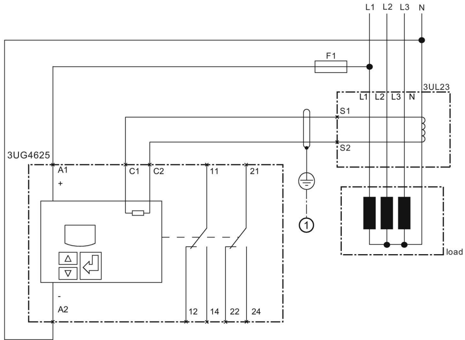
Figura 8-1 Ejemplo de circuito 3UG4625 con 3UL23
