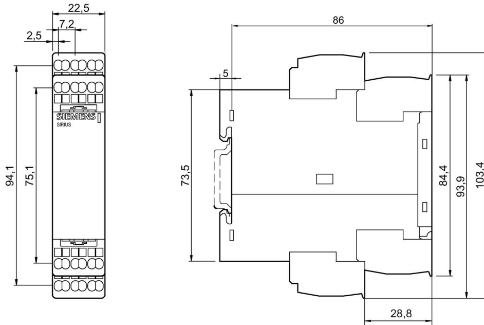
Figura C-22 Relés de monitoreo 3UG4. con 4 bornes de conexión de resorte
