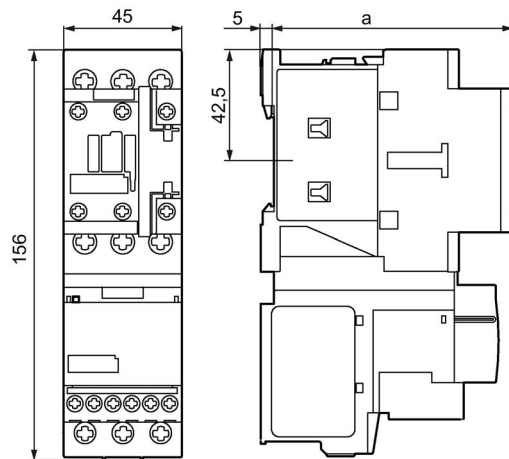
Figura C-5 3RR2.42-1A.30 con contactor
