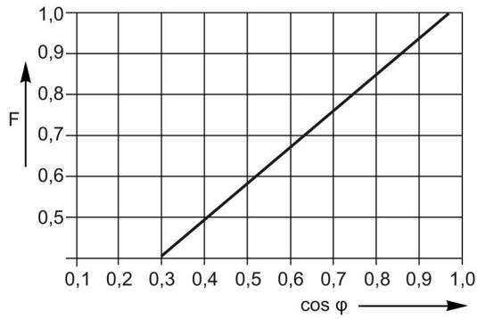
Figura 9-18 Factor de reducción F con carga AC inductiva
