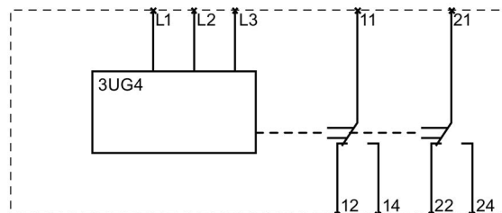
Figura 6-1 3UG4614
