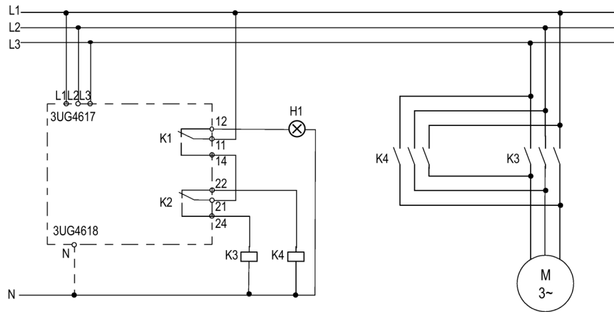
Figura 6-2 3UG4617/3UG4618 Corrección de fase automática
