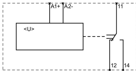
Figura 10-3 3UG4633
