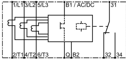
Figura 4-6 1 contacto conmutado, trifásico
