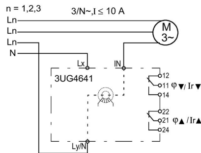
Monitoreo de corriente activa y cos phi para motores trifásicos (con neutro)
