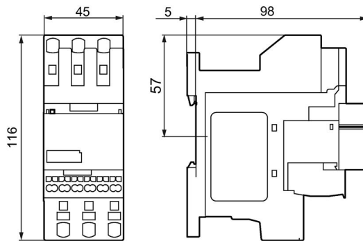
Figura C-8 3RR2.42-2A.30 con soporte de conexión para instalación independiente
