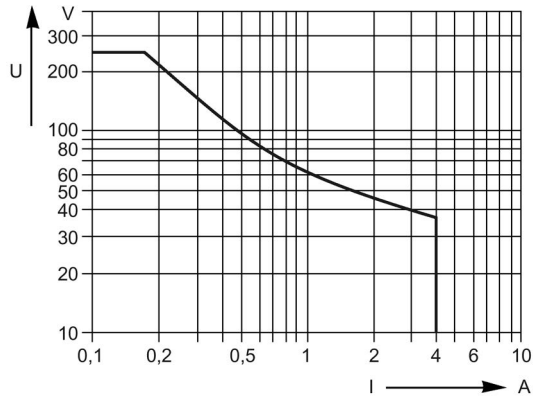
Figura 9-5 Carga DC (ohmica)
