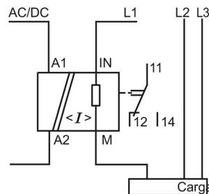
3UG462...-AW30 Modo trifásico
