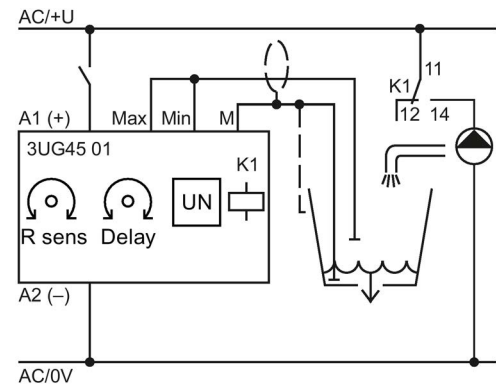
Regulación de un solo nivel
