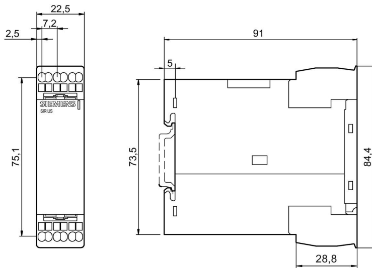
Figura C-18 Relés de monitoreo 3UG4. con 2 bornes de conexión de resorte
