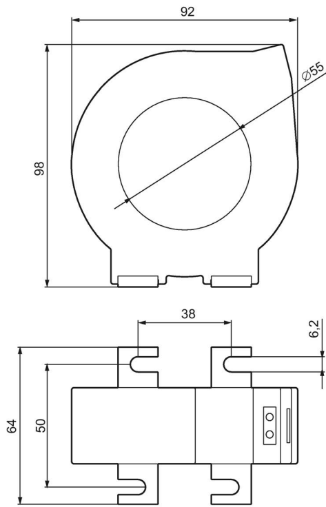
Figura 13-10 3UL2303-1A
