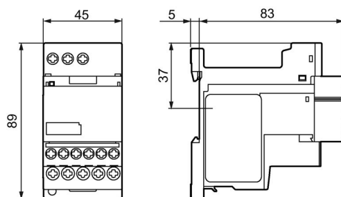
Figura C-2 3RR2.41-1A.30 con soporte de conexión para instalación independiente
