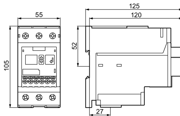
Figura C-14 3RR2243-1F.30 con soporte de conexión para instalación independiente
