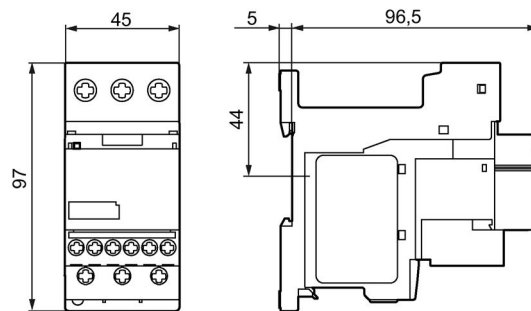
Figura C-6 3RR2.42-1A.30 con soporte de conexión para instalación independiente
