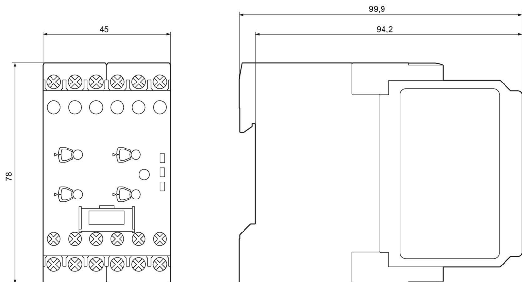
Figura C-24 Relé de monitoreo de aislamiento 3UG4583-1CW30
