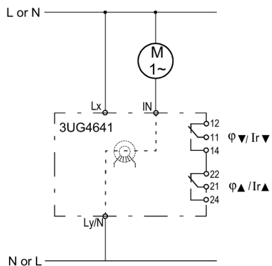
Figura 11-1 Monitoreo de corriente activa y cos phi para motores monofásicos
