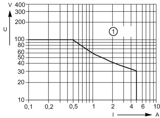
Figura 9-17 Carga DC (óhmica)
