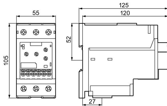
Figura C-10 3RR2143-1A.30 con soporte de conexión para instalación independiente
