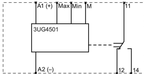
Relé de monitoreo de nivel de llenado 3UG4501-.A.30
