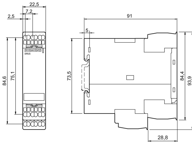
Figura C-20 Relés de monitoreo 3UG4. con 3 bornes de conexión de resorte
