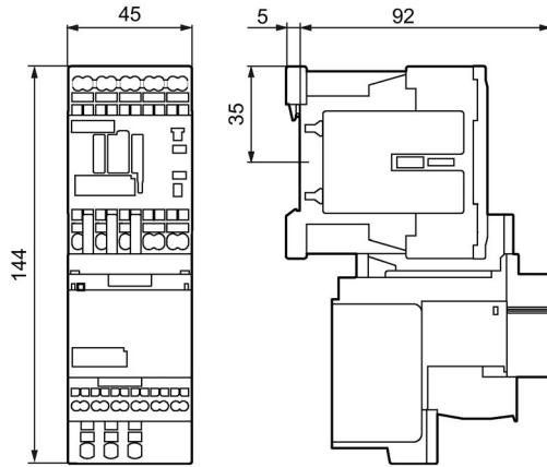
Figura C-3 3RR2.41-2A.30 con contactor
