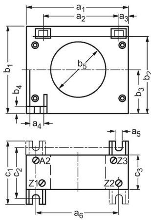
Figura 13-6 Transformador sumador de corriente 3UL22
