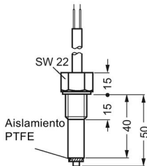
Figura 13-5 Electrodo de varilla monopolar 3UG3207-1C
