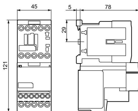
Figura C-1 3RR2.41-1A.30 con contactor
