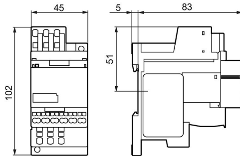
Figura C-4 3RR2.41-2A.30 con soporte de conexión para instalación independiente
