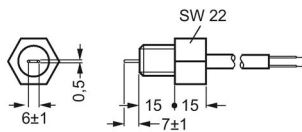
Figura 13-4 Electrodo de arco monopolar 3UG3207-1B
