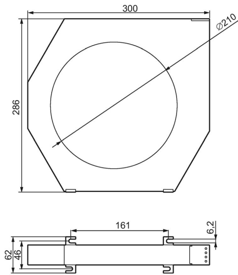
Figura 13-14 3UL2307-1A
