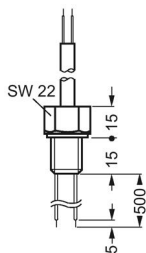
Figura 13-2 Electrodo de alambre bipolar 3UG3207-2A
