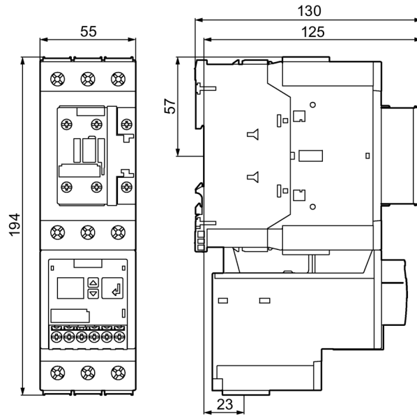
Figura C-13 3RR2243-1F.30 con contactor
