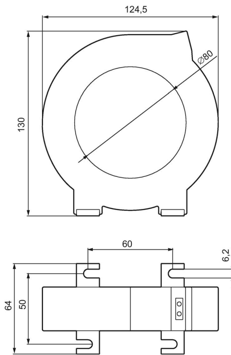
Figura 13-11 3UL2304-1A
