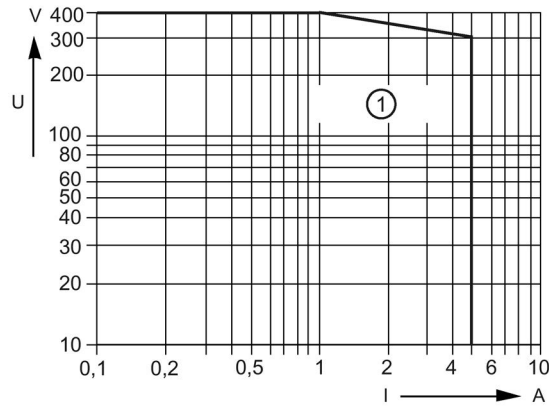
Figura 9-16 Carga AC (óhmica)
