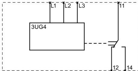
Relé de monitoreo de red 3UG4511-B..
