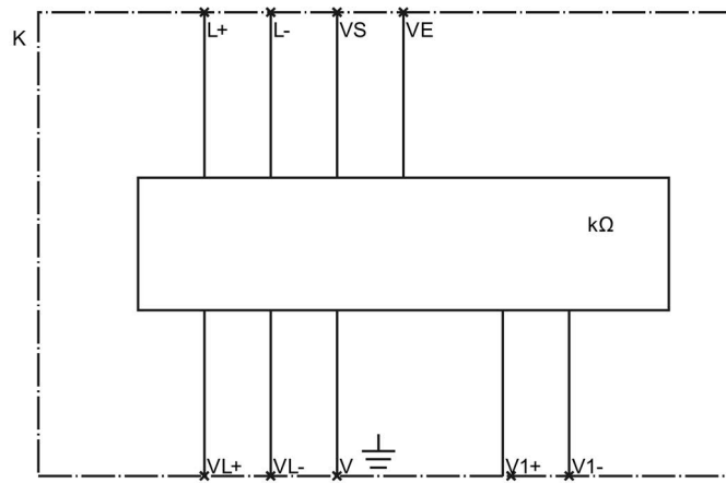
Figura 13-15 Relé de monitoreo de aislamiento 3UG4983-1A
