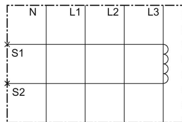
Figura 13-8 Transformador de corriente diferencial 3UL23
