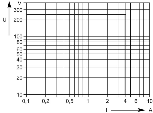
Figura 9-4 Carga AC (ohmica)
