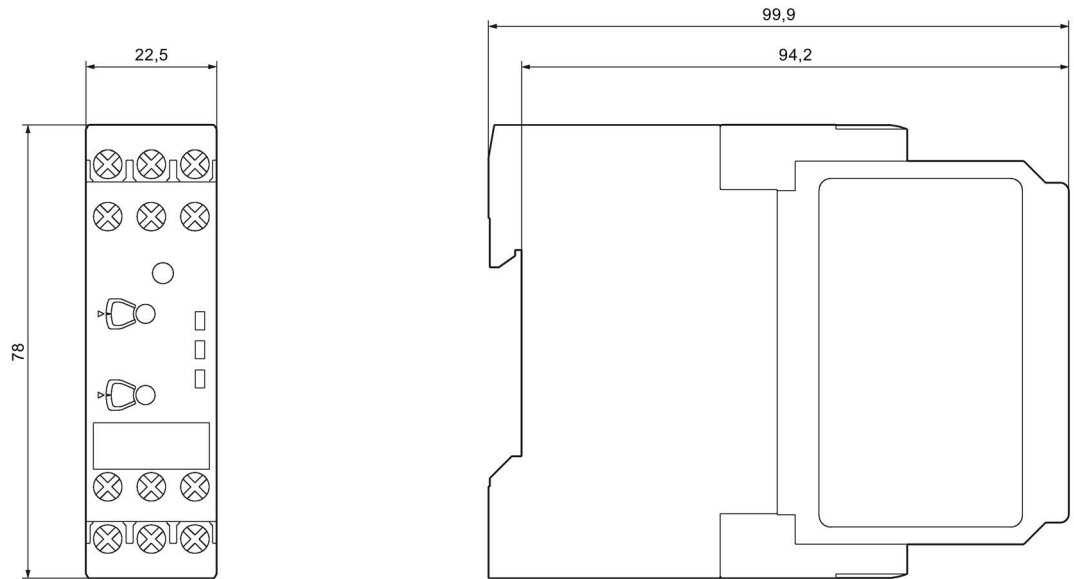
Figura C-23 Relés de monitoreo de aislamiento 3UG4581-1AW30/3UG4582-1AW30
