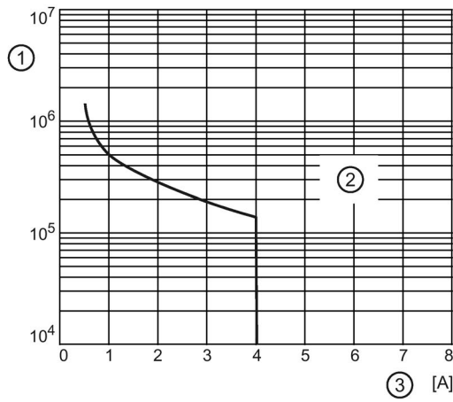
Figura 9-6 Factor de reducción F con carga AC inductiva
