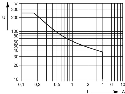
Figura 9-13 Carga DC (ohmica)
