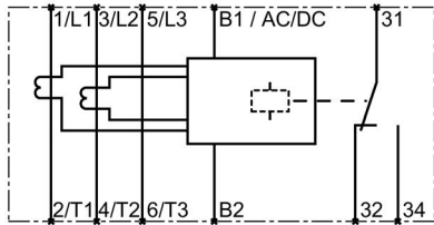
Figura 4-3 1 contacto conmutado, bifásico
