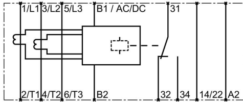
Figura 4-2 1 contacto conmutado, bifásico
