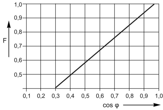
Figura 9-14 Factor de reducción F con carga AC inductiva
