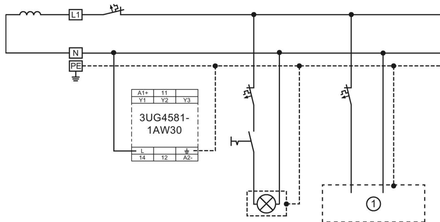
Figura 9-2 Vigilancia de falla a tierra/defectos de aislamiento en una red AC IT de 2 conductores
