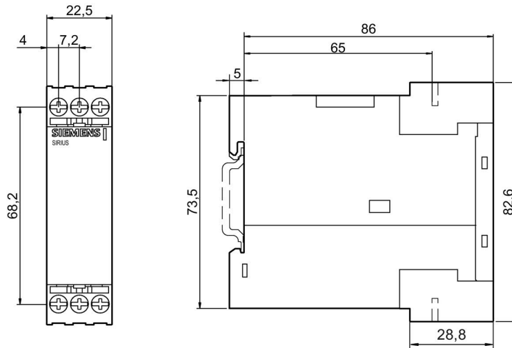
Figura C-17 Relés de monitoreo 3UG4. con 2 bornes de conexión de tornillo
