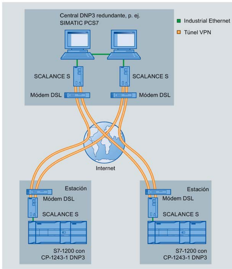
Figura 1-3 Ejemplo de configuración con central DNP3 redundante
