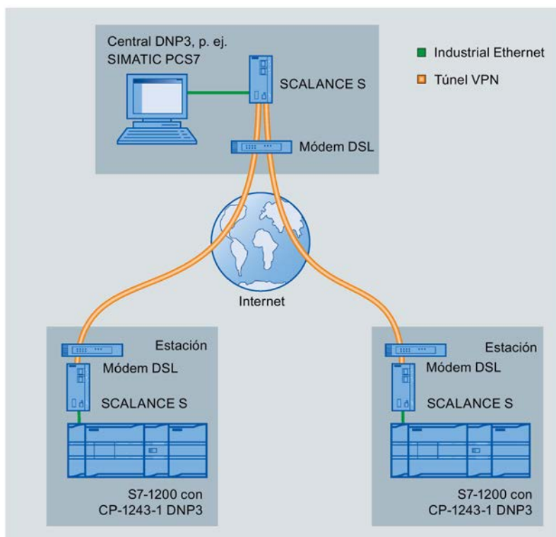
Figura 1-2 Ejemplo de configuración con conexiones vía Internet
