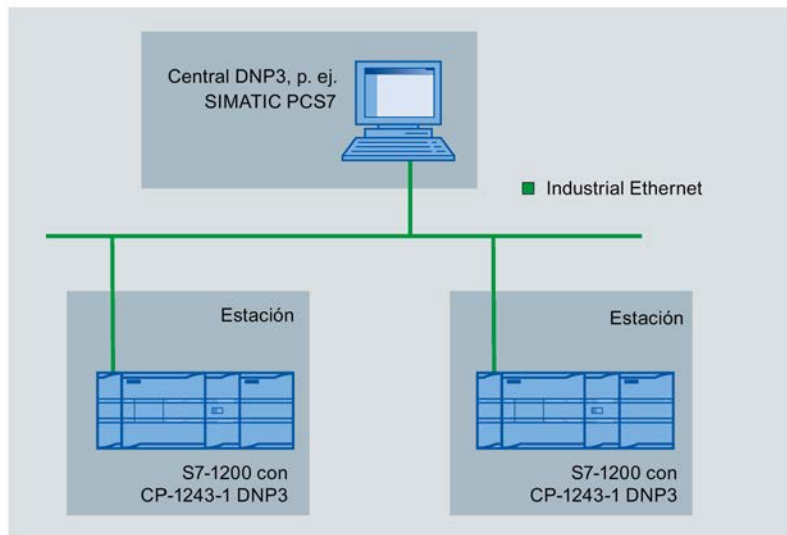
Figura 1-1 Ejemplo de configuración con central de supervisión simple y estaciones en una subred IP
