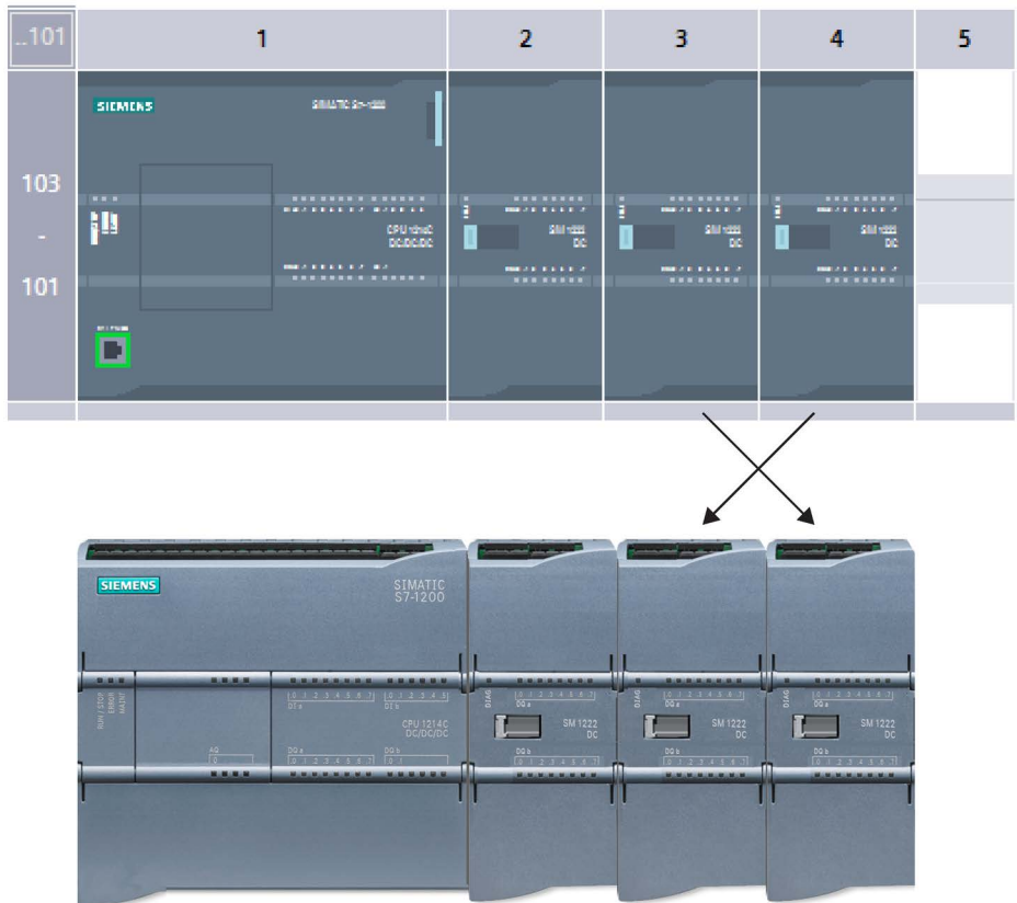
Figura 6-3 Configuración del dispositivo comparado con la instalación real con módulos intercambiados en los slots 3 y 4
