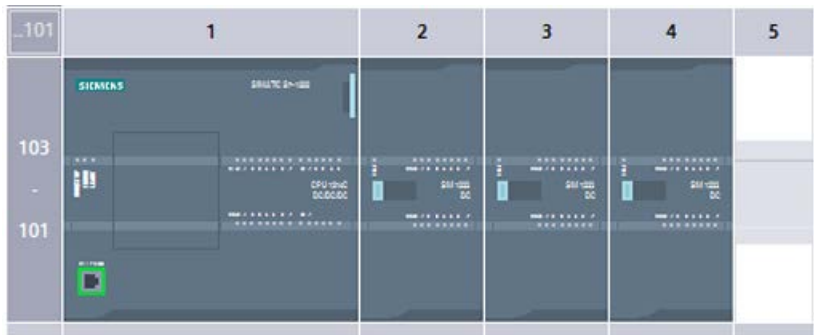
Figura 6-1 Configuración del dispositivo para una instalación máxima
