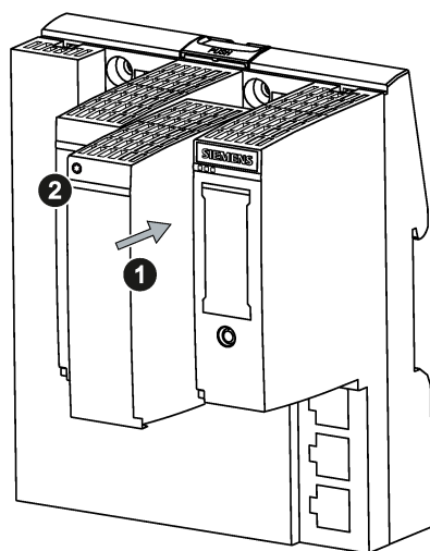
Figura 4-3 Montar un adaptador de bus
