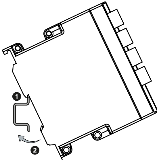
Figura 4-1 Montaje sobre un perfil DIN (35 mm)
