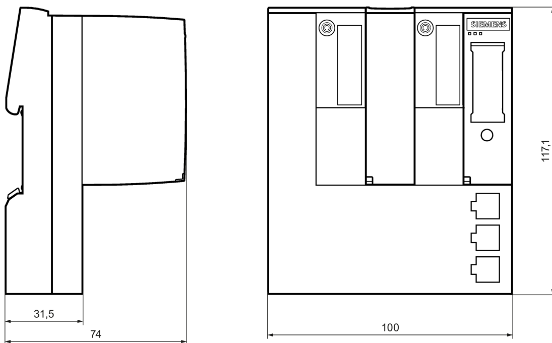
Figura A-9 Plano acotado del SCALANCE XF204-2BA IRT
