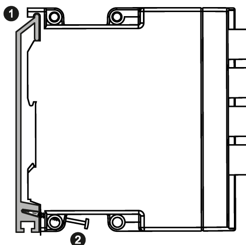
Figura 4-2 Montaje sobre un perfil soporte SIMATIC S7-300
