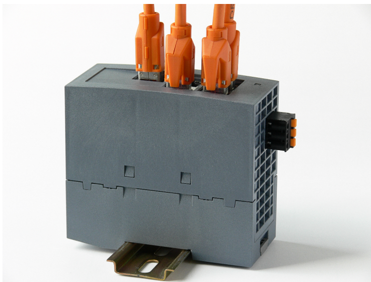
Figura 5-2 SCALANCE XB-000 montado sobre el perfil DIN simétrico (35 mm)
