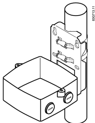
Figura 4-7 Montaje en tubería - vertical
