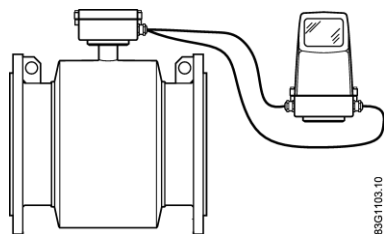
Figura 4-2 Instalación remota
