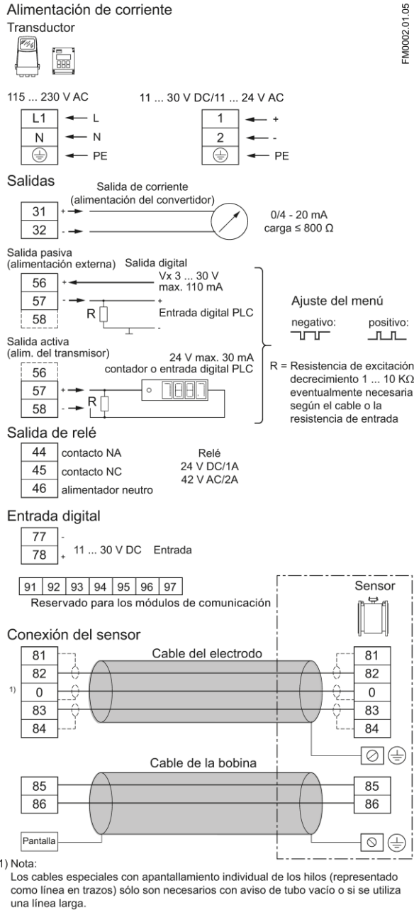
Figura 5-1 Diagrama de cableado
