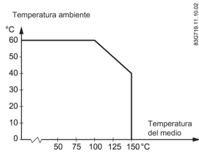
Figura 4-4 Versiones estándar, sin pantalla y SV
