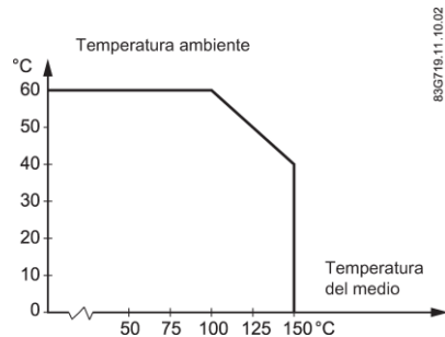
Figura 4-5 Versión CT
