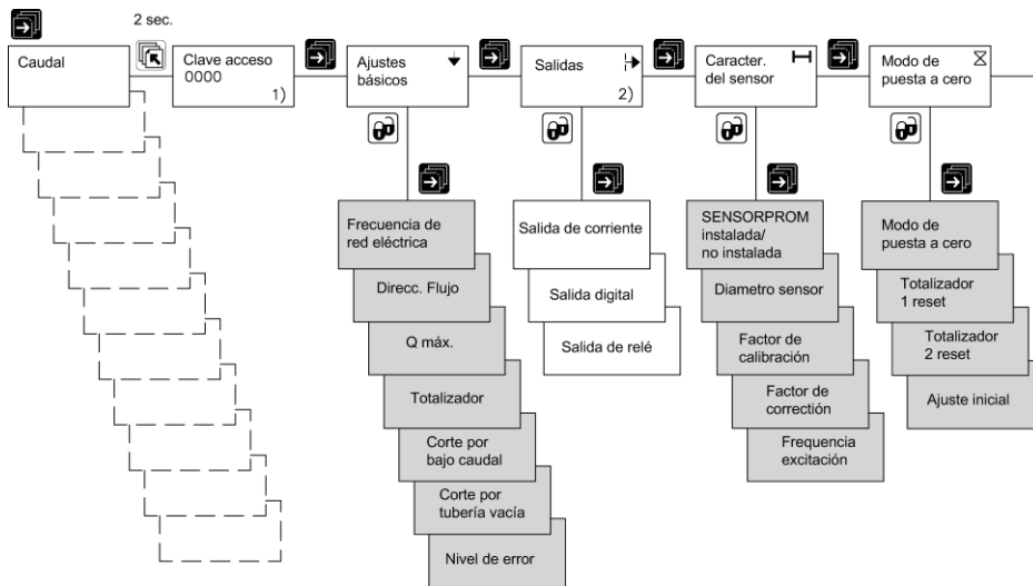
Figura A-1 Vista general del MAG 5000 CT y MAG 6000 CT (parte 1)
