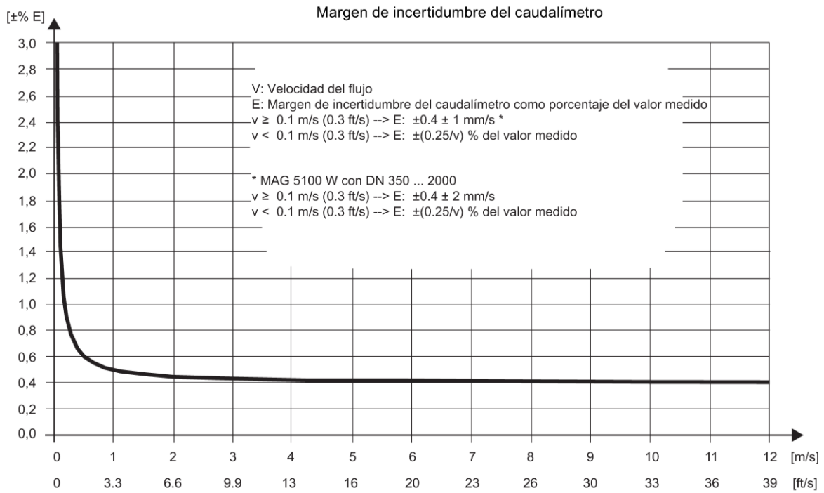
Figura 11-1 MAG 5000 con MAG 1100, MAG 1100 F, MAG 5100 W, MAG 3100 y MAG 3100 P y MAG 6000 con MAG 1100 (PFA), MAG 1100 F (PFA)
