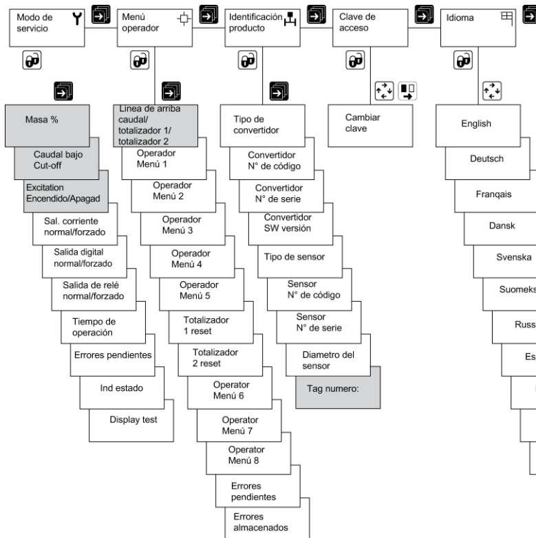
Figura A-1 Vista general del MAG 5000 CT y MAG 6000 CT (parte 1)
