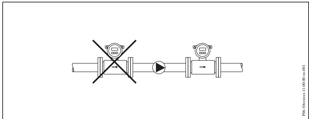
Рис. 6: Установка насосов
