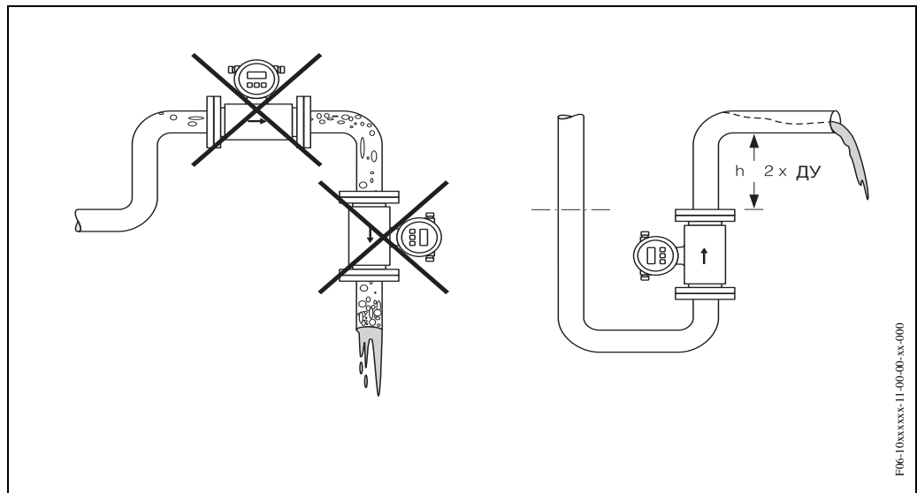
Рис. 5: Место монтажа
